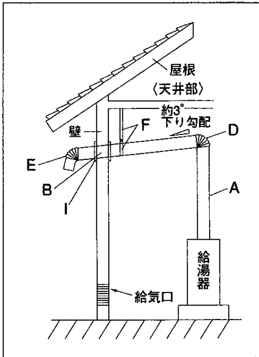
強制排気式取付施工図
