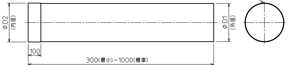
拡管タイプ
