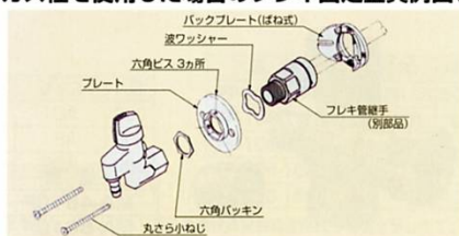
現行ガス栓を使用した場合のフレキ固定金具例図(一口用)
