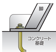
アンカーボルト
