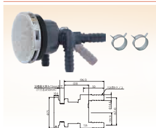
15Aタケノコ式LS兼用
