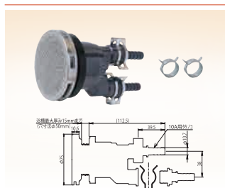
クイック10Aタケノコ式S
