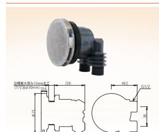
オスネジ式L
