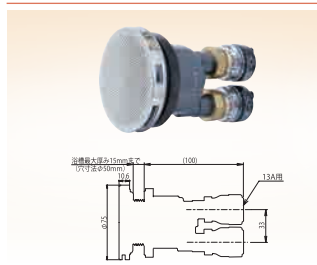
13Aワンロック式S
