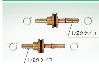
ST15型 1/2タケノコ×1/2タケノコ(S)
